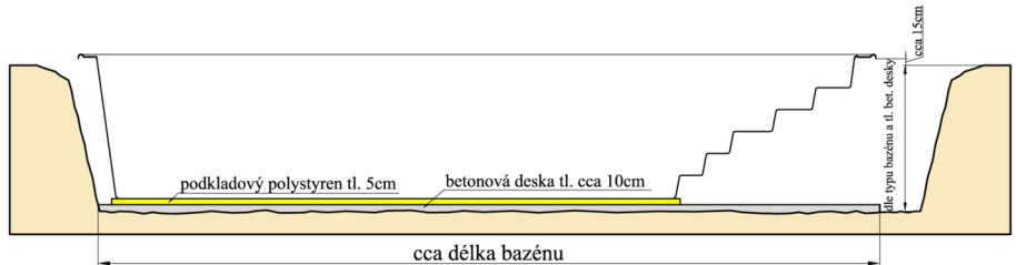
podélný řez výkopem - bazén je usazen na podkladový polystyren a částečně povysazen nad terén
