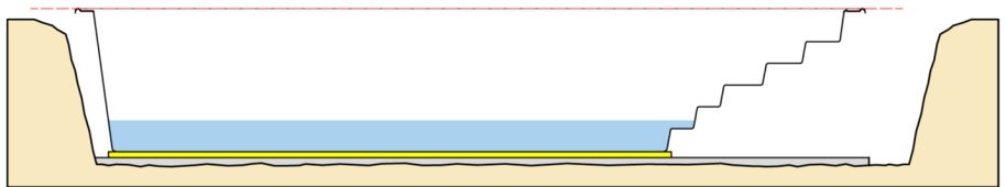
kontrola rovinnosti límce - korekce v případě pokleslého límce se provádí podepřením a srovnáním daného místa
