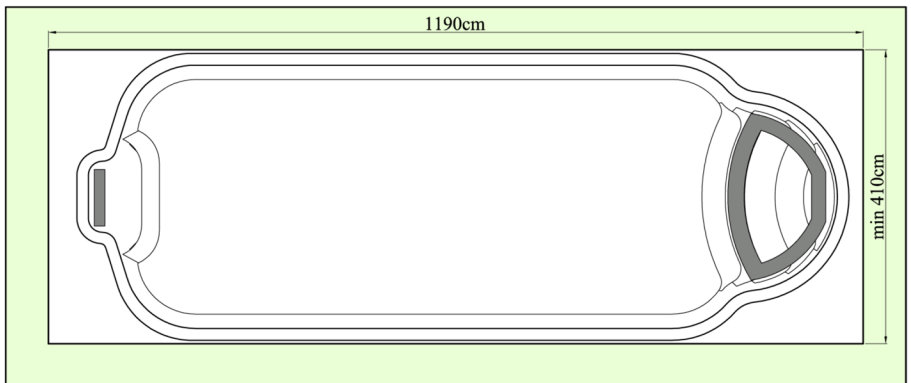
schéma podezdění bazénového schodiště a sedáku
