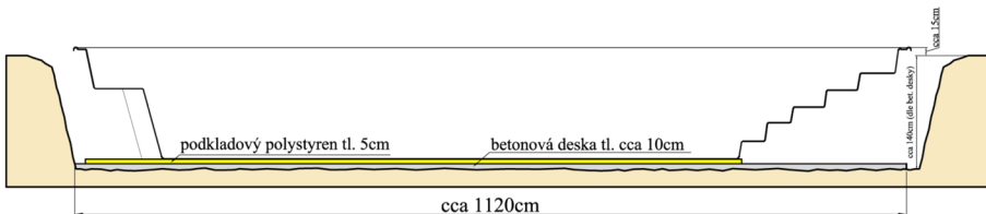
podélný řez výkopem - bazén je usazen na podkladový polystyren a částečně povysazen nad terén
