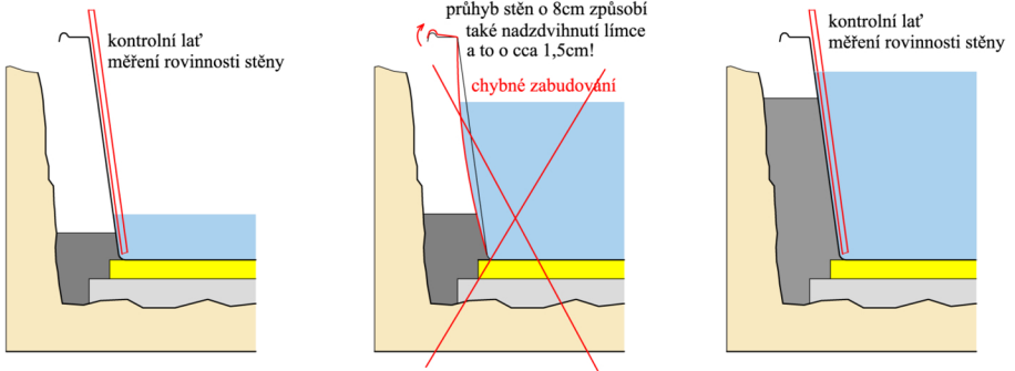
kontrola rovinnosti stěn ve svislém směru
