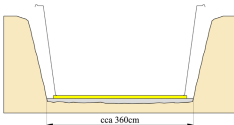
příčný řez výkopem - šířka betonové desky cca 360cm
